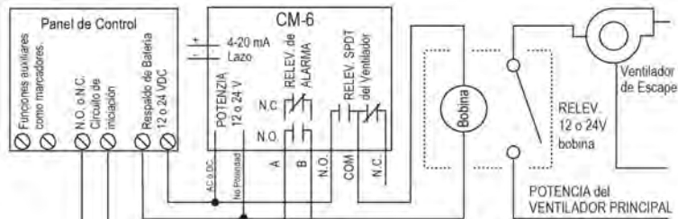
Conexión típica CM-6 y panel de control
